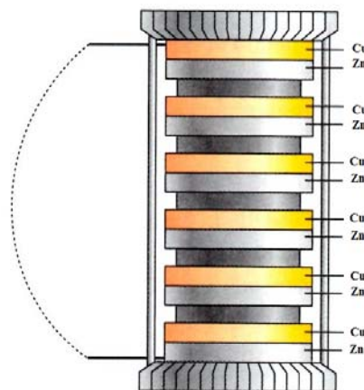
fig. 1.2: Pila a colonna
